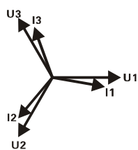
三相四线向量图
