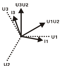
三相三线向量图
